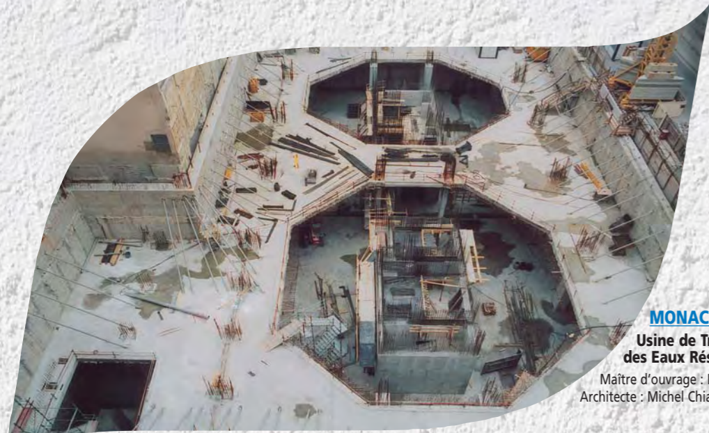
Soutènement avec dalle haubanée Conception (brevet) et direction travaux pour Solétanche
